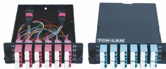
SLOT MPO PER CASSETTO OTTICO
